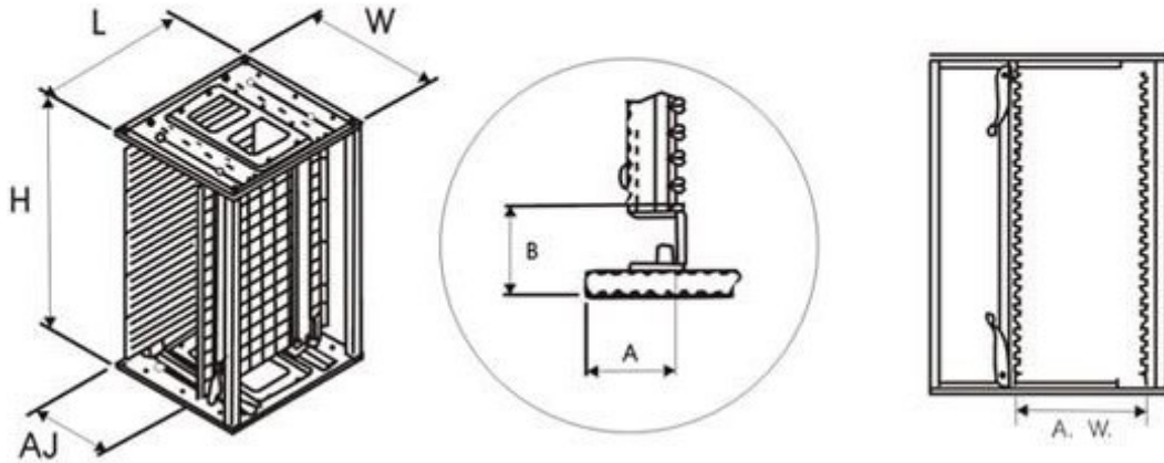
收集箱（架）尺寸示意 Magazine Dimensions
